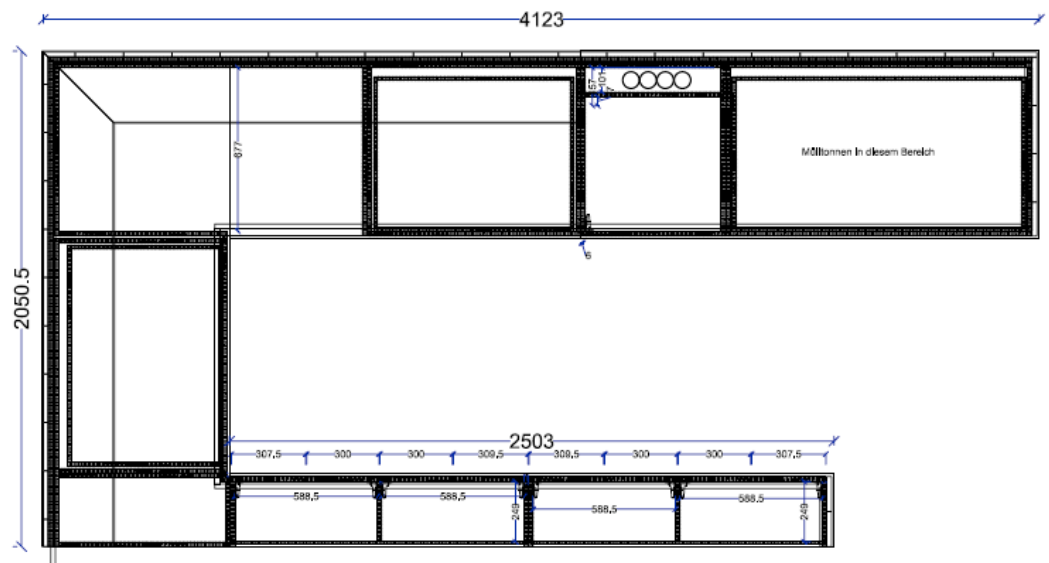
Draufsicht Theke
